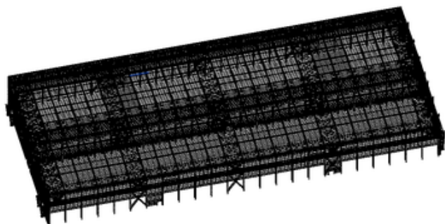
（图为Taka1模型深化后钢结构模型）
