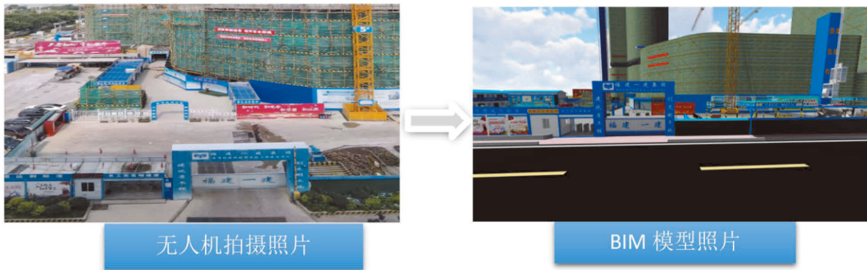
图 1 现场照片与场地模型照片对比
