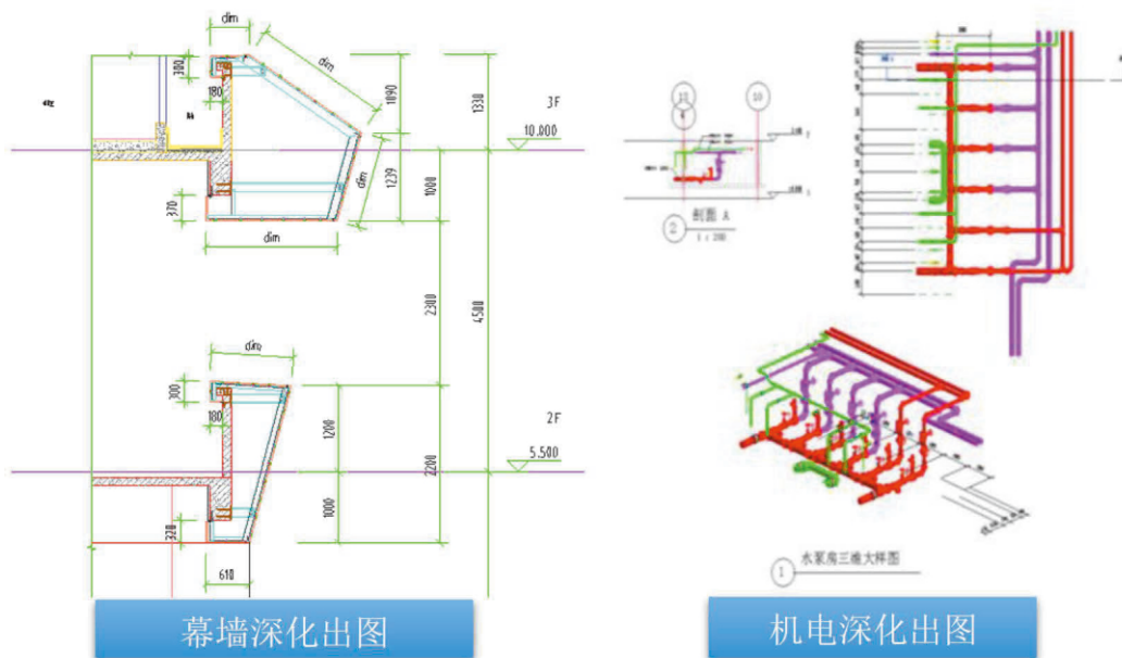
图 3 幕墙深化与机电泵房深化出图
