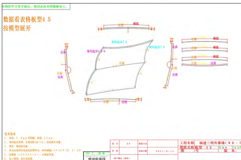
图5 铝单板数据加工图
